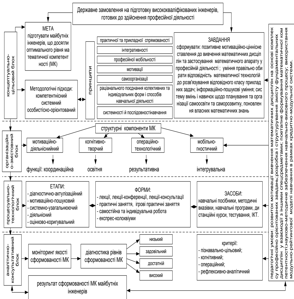
Рис.1 – Структурна модель формування математичної компетентності майбутніх інженерів
